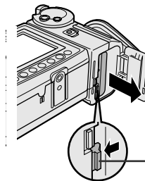
Фиксатор аккумулятора
