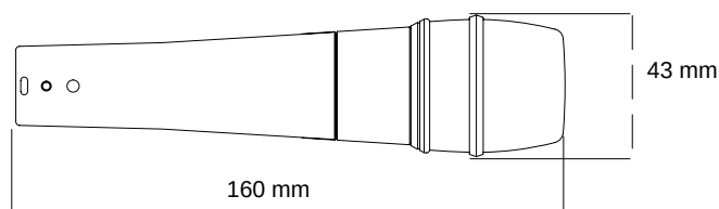
ГАБАРИТЫ
