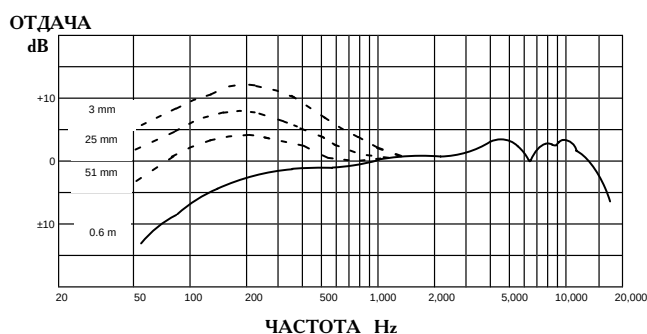
ЧАСТОТНАЯ ХАРАКТЕРИСТИКА
