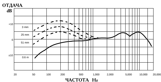
ЧАСТОТНАЯ ХАРАКТЕРИСТИКА
