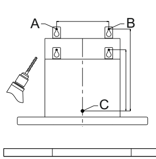
نموذج التركيب
