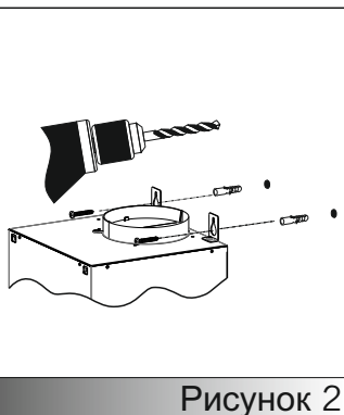
Шаблон монтажа
