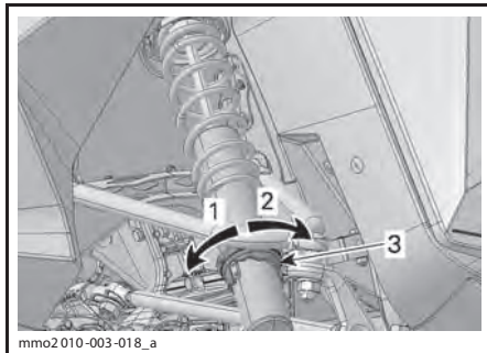
РЕГУЛЯТОР КУЛАЧКОВОГО ТИПА — АМОРТИЗАТОР MOTION CONTROL
