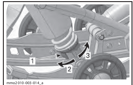
РЕГУЛЯТОР КУЛАЧКОВОГО ТИПА — АМОРТИЗАТОР MOTION CONTROL
