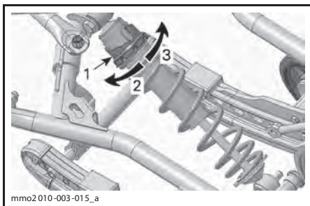
РЕГУЛЯТОР КУЛАЧКОВОГО ТИПА — АМОРТИЗАТОР НРГ™
