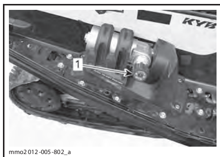
ТИПОВОЙ ВАРИАНТ — MOTION С ВЫНОСНЫМ РЕГУЛИРОВОЧНЫМ ЭЛЕМЕНТОМ — ПРАВАЯ СТОРОНА
