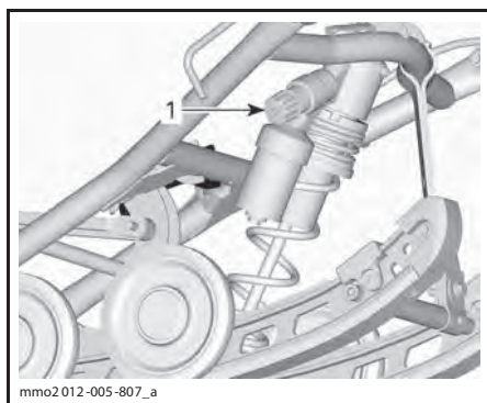
1. Рукоятка регулировки демпфирования хода сжатия центрального амортизатора
