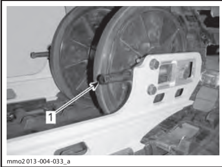
1. Левый регулировочный винт
