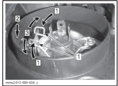
Шаг 1: Сжать с обеих сторон Шаг 2: Нажать вниз, чтобы освободить Шаг 3: Освободить обе стороны 1. Защёлка
