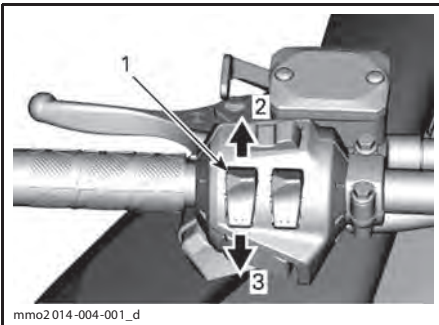
ИЗМЕНЕНИЕ ИНТЕНСИВНОСТИ ОБОГРЕВА
