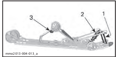
tMOTION — РЕГУЛИРУЕМЫЕ КОМПОНЕНТЫ
