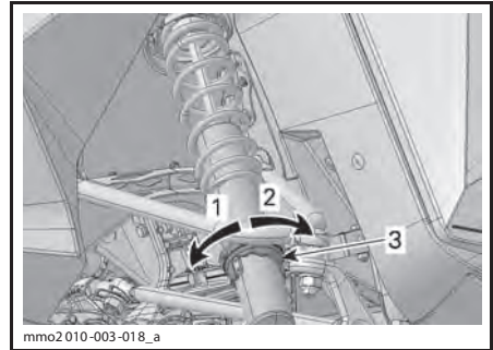
РЕГУЛЯТОР КУЛАЧКОВОГО ТИПА — АМОТИЗАТОР MOTION CONTROL
