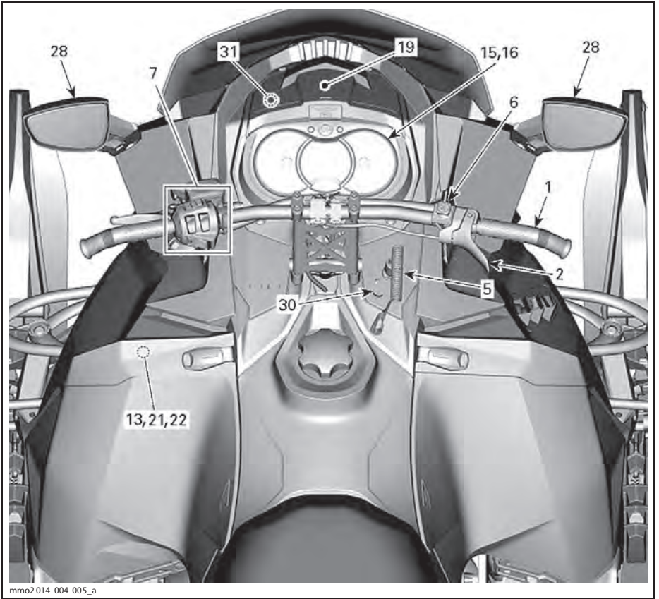
ТИПОВОЙ ВАРИАНТ — МОДЕЛИ MX Z, RENEGADE И GSX LE
