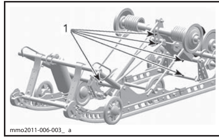
1. Пресс-масленки
