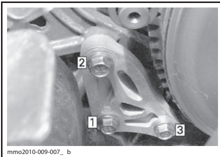
ПОСЛЕДОВАТЕЛЬНОСТЬ ЗАТЯЖКИ
