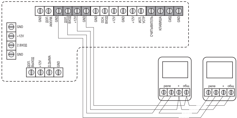
Подключение датчиков к дополнительному входу
