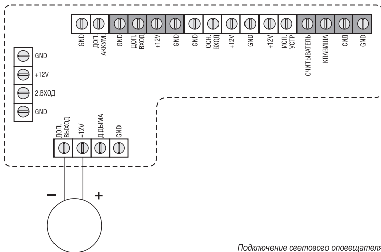
Подключение светового оповещателя
