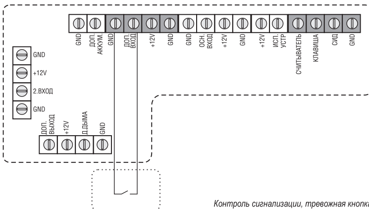
Контроль сигнализации, тревожная кнопка
