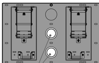
Aukko kaapeleita varten (toinen kahdesta)
