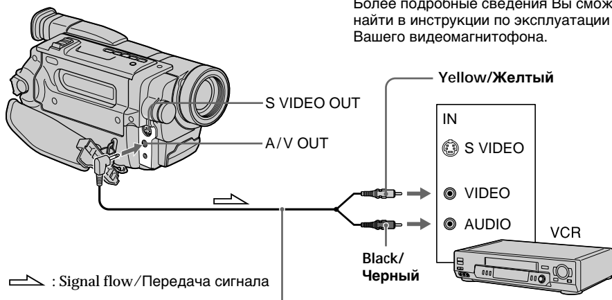
A/V connecting cable (supplied)/ Соединительный кабель аудио/видео (прилагается)
