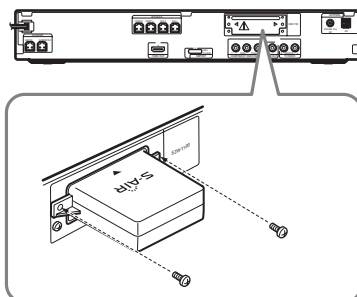
Задняя панель устройства
