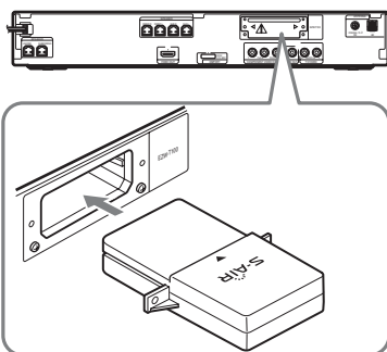
Задняя панель устройства
