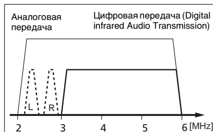
Рис. 1 Спектр сигнала при передаче по технологии Digital Infrared Audio Transmission
