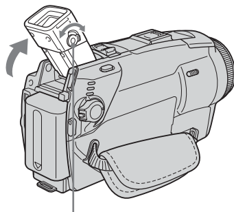
Рычаг регулировки объектива видоискателя
