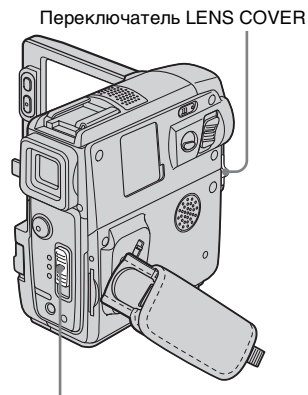
Переключатель POWER
