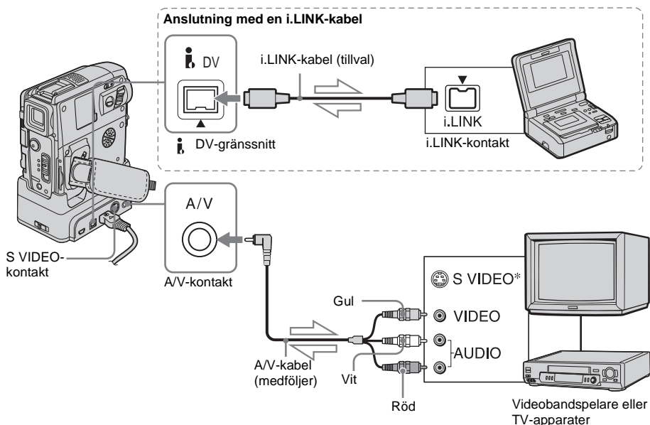
Signalflöde
