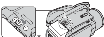
Кнопка фиксатора батареи BATT
