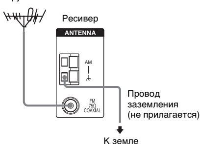
Наружная антенна FM
