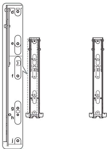
Положение винтов
