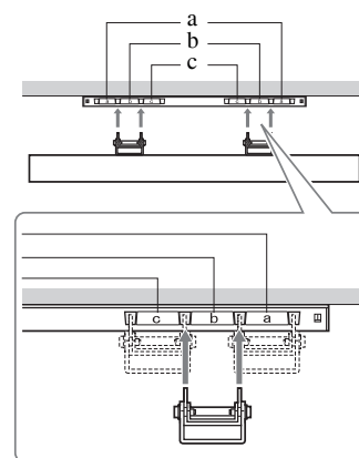
Расположение скоб
