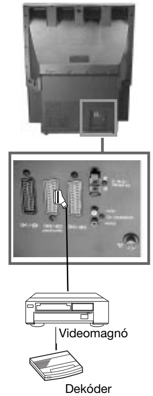
A projekciós TV hátlapja
