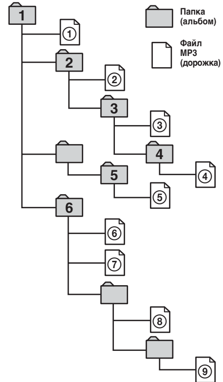
Дерево 1 Дерево 2 Дерево 3 Дерево 4 Дерево 5 (корневое)
