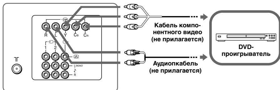
Задняя панель ТВ
