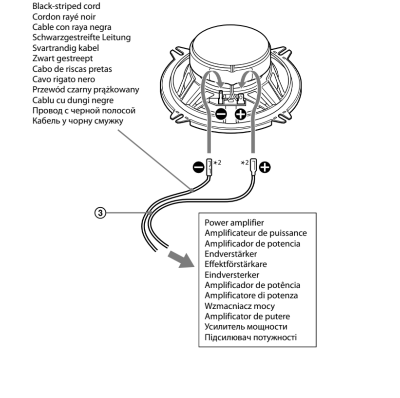
*1 White cord — Left speaker Gray cord — Right speaker *2 Cordon blanc — Haut-parleur gauche Cordon gris — Haut-parleur droit *3 Cable blanco — Altavoz izquierdo Cable gris — Altavoz derecho *4 Weißes Kabel — Linker Lautsprecher Graues Kabel — Rechter Lautsprecher *5 Vir kabel — Vänster högtalare Grå kabel — Höger högtalare *6 Vir snood — LinkerLuidspreker Gris snood — RechterLuidspreker
