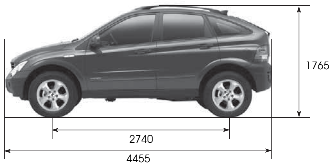
Вид сбоку
