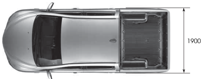
Вид сверху
