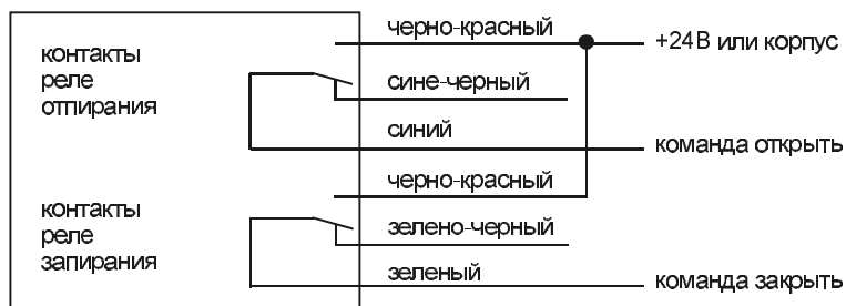
Схема подключения к двухпроводным приводам системы запирания
