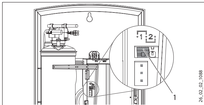
1 Кодировочный разъем
