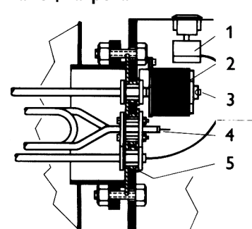
Фланец нагрева
