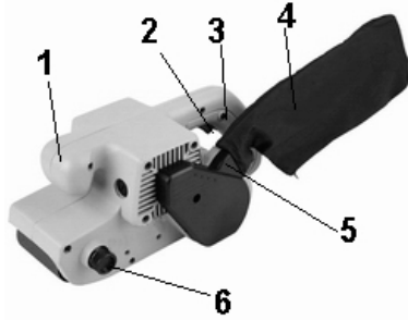
Внешний вид BS8580
