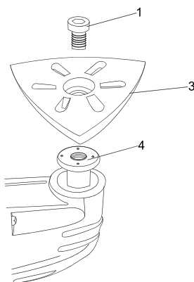
установка приспособления для полировки
