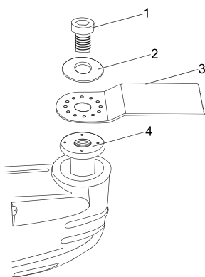
Установка ножа
