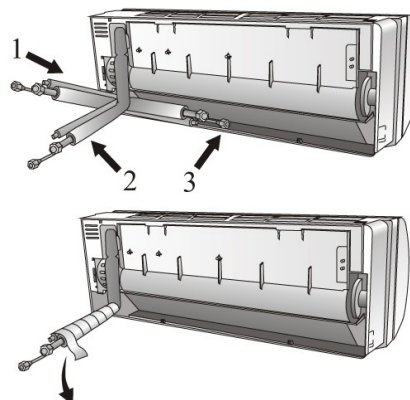
распрямление соединительной трубы
