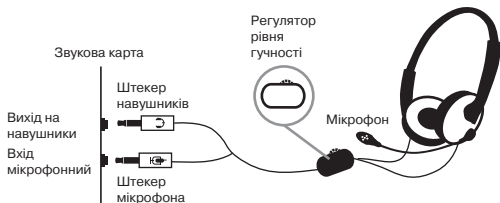
Мал. 1. Схема підключення
