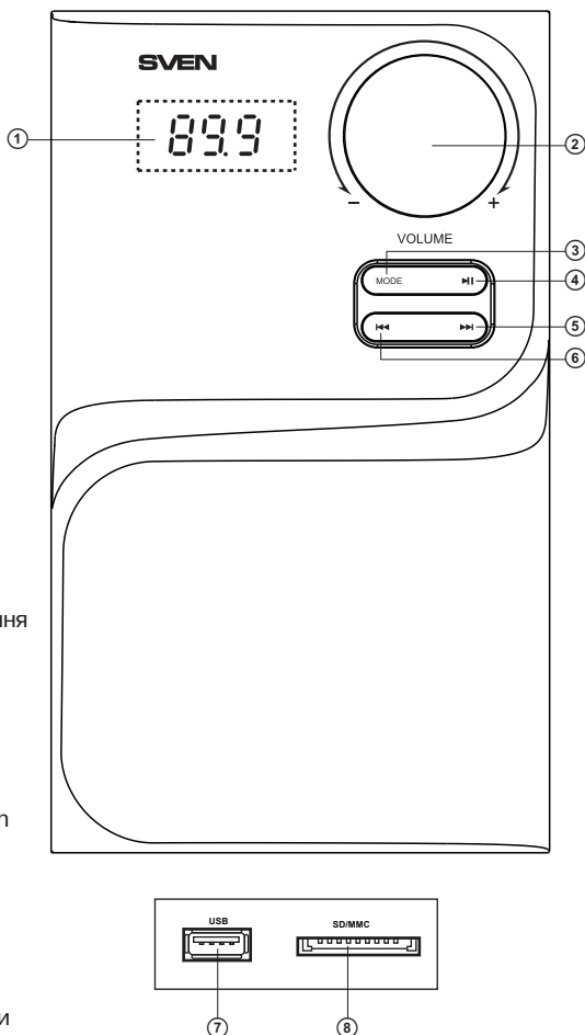
Мал. 1. Панель управління сабвуфера
