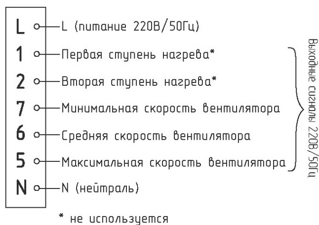
Рисунок 8-Назначение клемм пульты управления (IR03)
