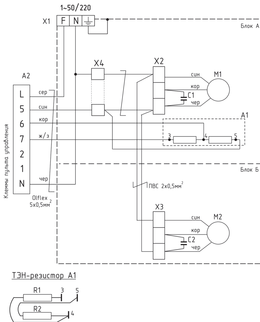
Рисунок 8-Назначение клемм пульты управления (IR03)
