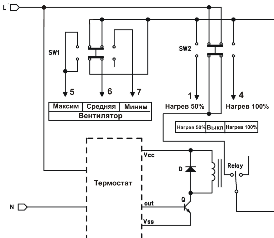
Рис. 6. Электрическая схема пульта управления
