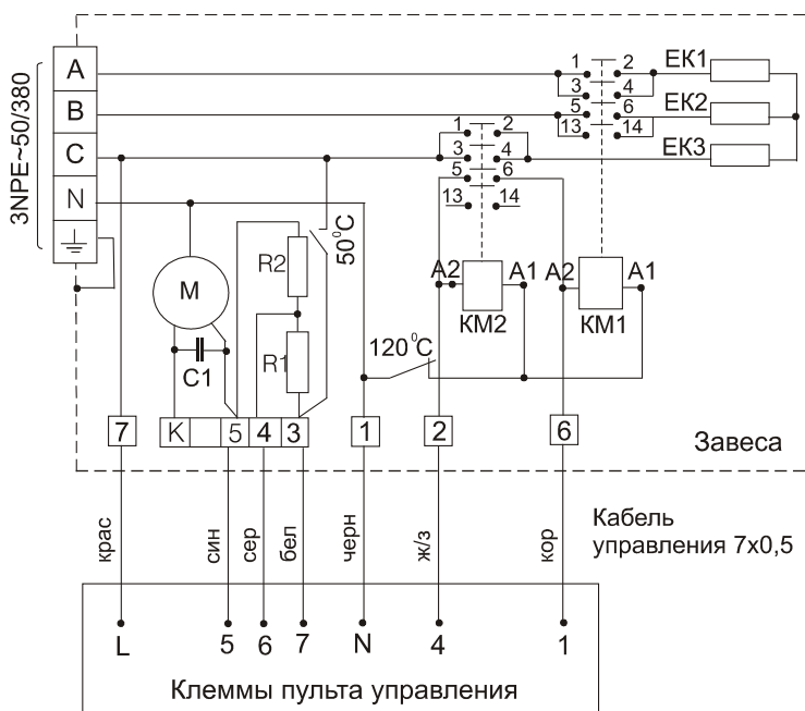
Рис. 2. Электрическая схема КЭВ-П302Е, КЭВ-П303Е
