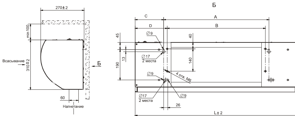
Рис. 8. Крепежные размеры
