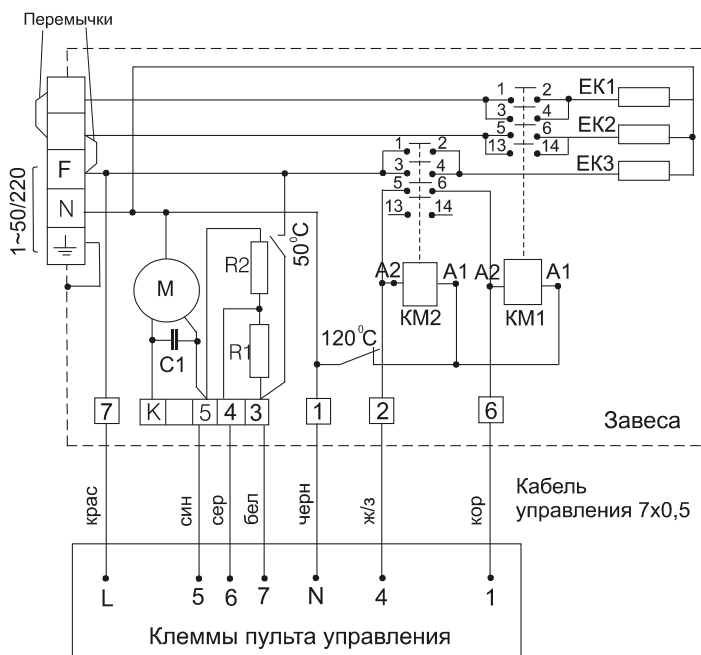
Рис. 1. Электрическая схема КЭВ-6П323Е
