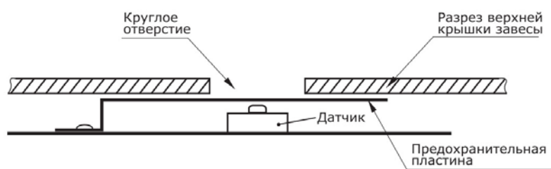
Рис. 9. Аварийный термовыключатель
