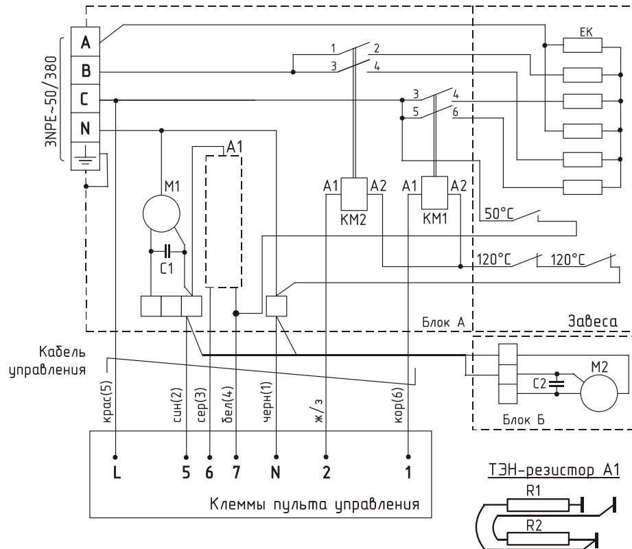
Рис. 4. Электрическая схема КЭВ-9П2020Е, КЭВ-12П2020Е
