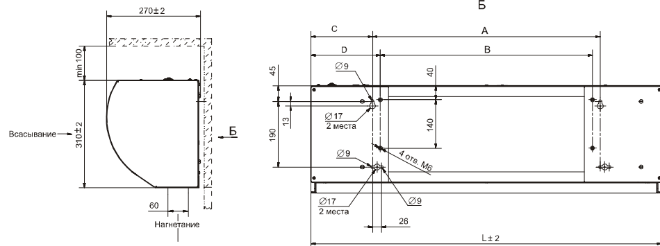
Рис. 5. Крепежные размеры КЭВ-П313А, КЭВ-П314А
