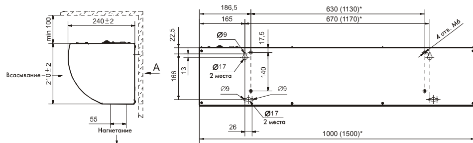
Рис. 4. Крепежные размеры КЭВ-П211А, КЭВ-П212А
