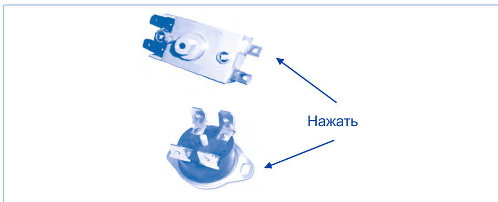
Рис. 4. Схема расположения кнопки термовыключателя
