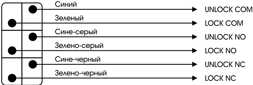
Схема подключения центрального замка
