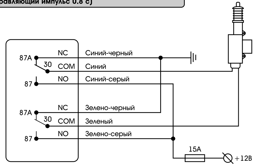
Схема подключения дополнительного электропривода (управляющий импульс 0.8 с)
