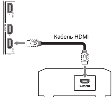
AV-усилитель, который поддерживает ARC
