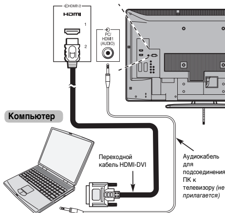
задняя панель телевизора
