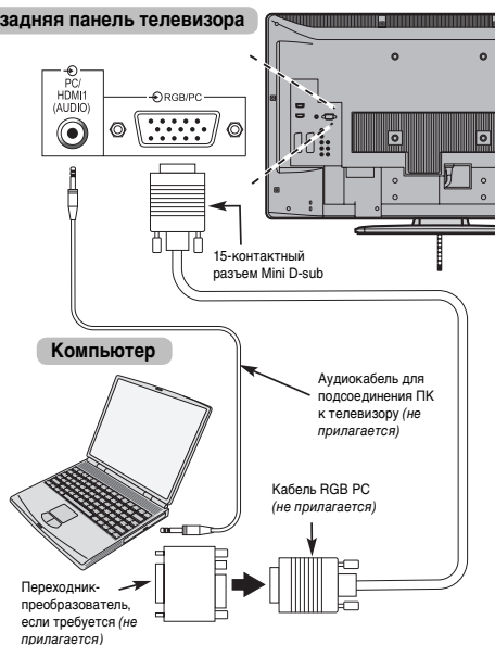
задняя панель телевизора
