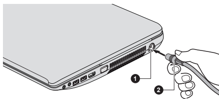
Рисунок 2-5 Подключение штекера вывода адаптера переменного тока к компьютеру (X70-A)
