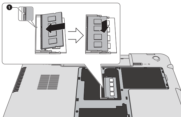
Рисунок 4-14 Установка модуля памяти
