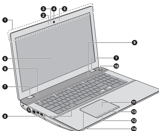
Рисунок 3-12 Вид компьютера спереди с открытой панелью дисплея (модели P70-A с сенсорным экраном)
