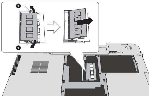
Рисунок 4-16 Удаление модуля памяти
