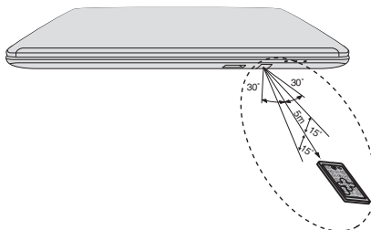
Рисунок 4-3 Радиус действия пульта дистанционного управления
