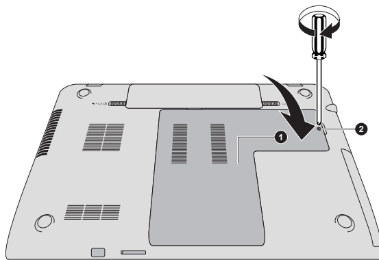
1. Крышка отсека модулей памяти 2. Винт
