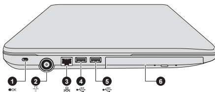
Рисунок 3-4 Левая сторона компьютера (X70-A)
