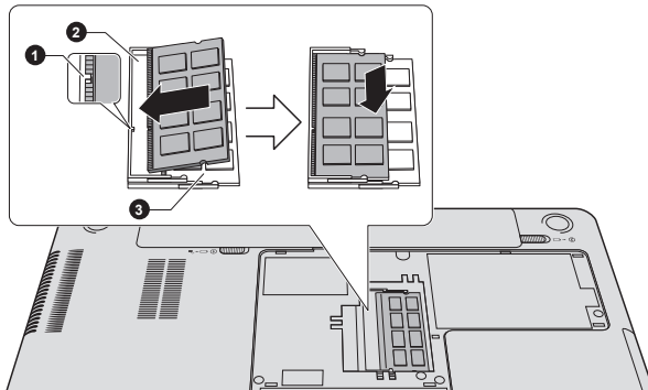
Рисунок 4-13 Установка модуля памяти
