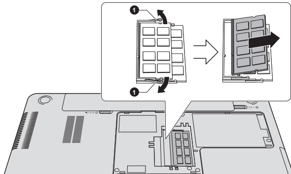
Рисунок 4-15 Удаление модуля памяти
