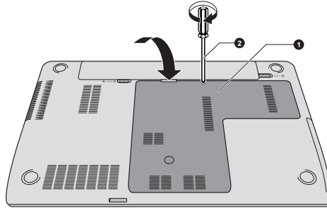
Рисунок 4-14 Установка крышки отсека модулей памяти
