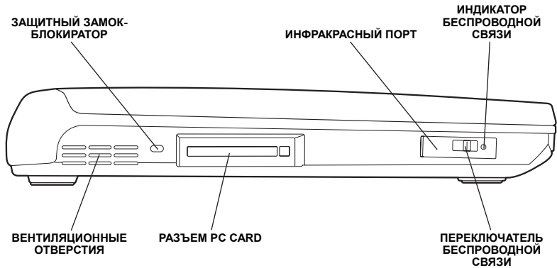
Левая сторона компьютера
