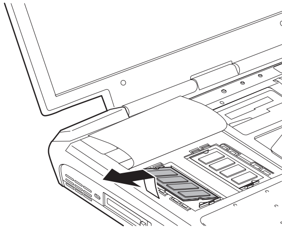
Удаляем модуль памяти
