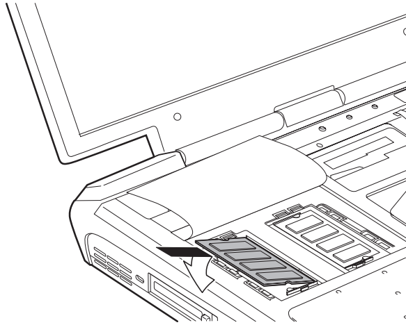
Устанавливаем модуль памяти
