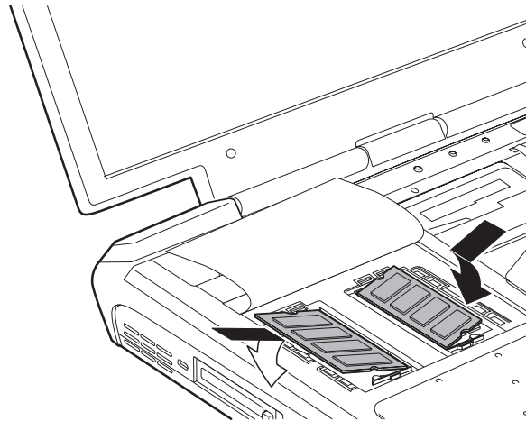
Устанавливаем два модуля памяти
