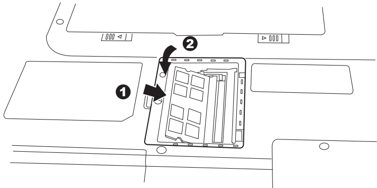
Установка модуля
