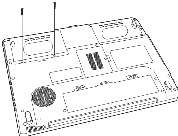
Снимаем крышку отсека для установки модулей памяти
