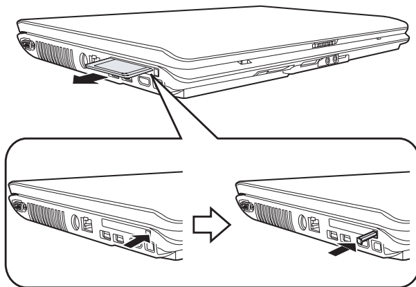
Удаление карты памяти Express Card
