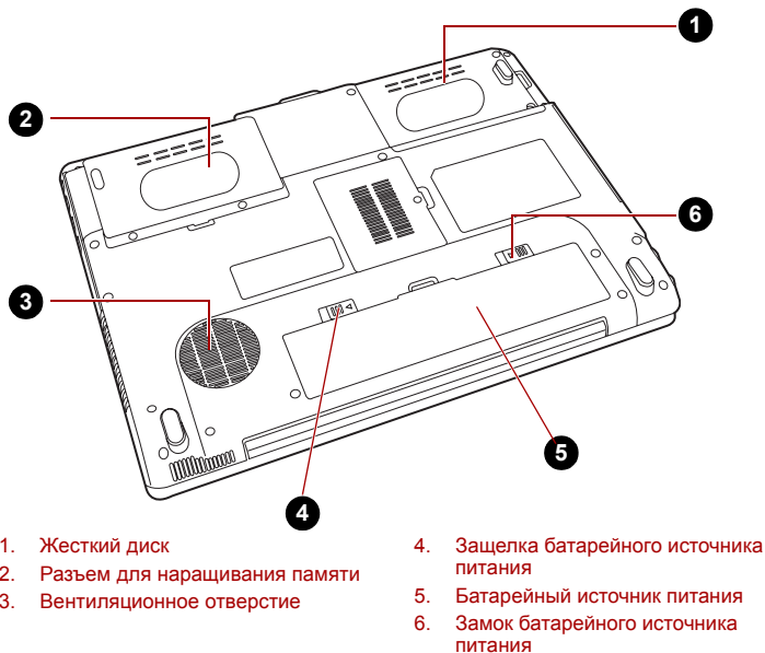
Нижняя сторона компьютера
