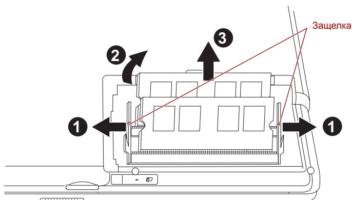
Удаление модуля памяти
