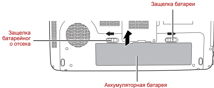
Высвобождение аккумуляторной батареи
