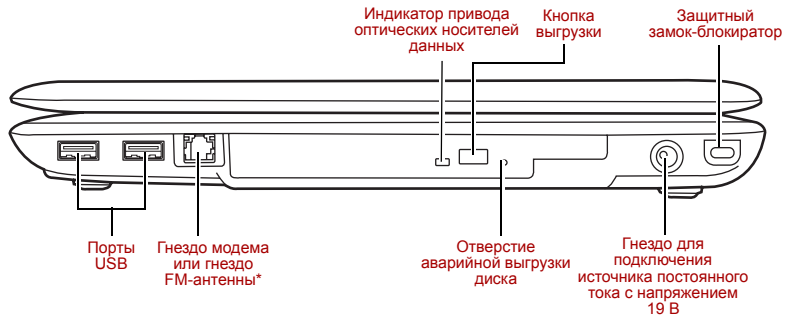
Вид компьютера справа
