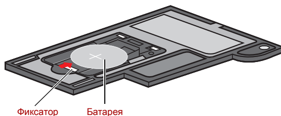
Установка батареек
