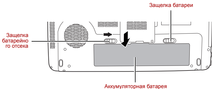
Закрепление аккумуляторной батареи
