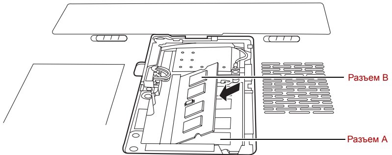
Установка модуля памяти.
