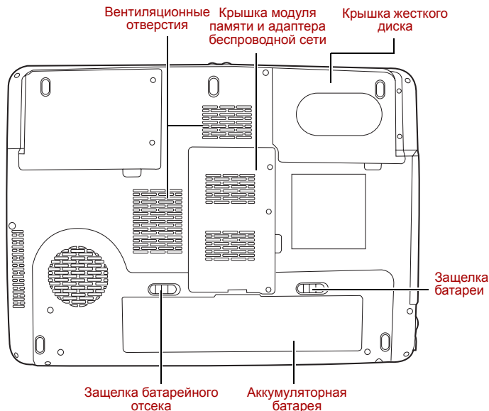
Вид компьютера снизу
