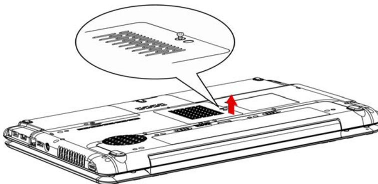
Рисунок 8-7 Снимаем крышку
