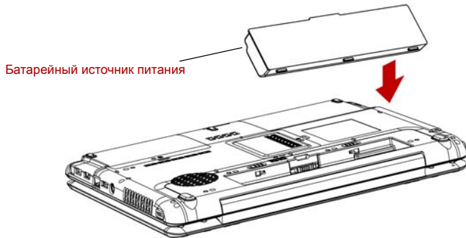
Рисунок 6-3 Установка батарейного источника питания
