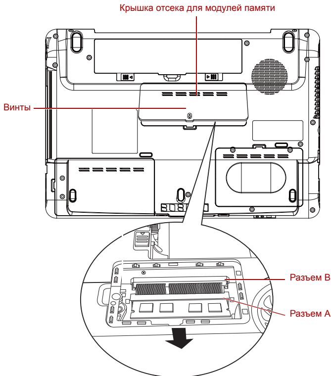
Рисунок 8-6 Снимаем крышку отсека для модулей памяти
