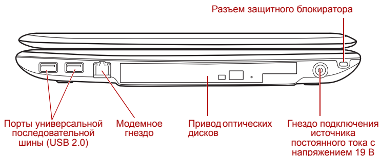
Рисунок 2-3 Вид компьютера справа
