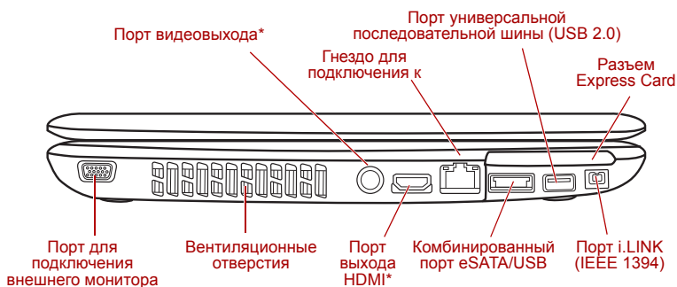
Рисунок 2-2 Вид компьютера слева
