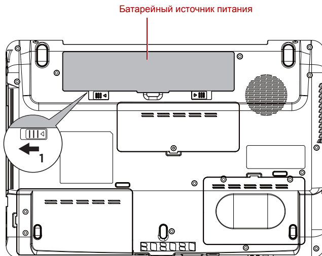
Рисунок 6-1 Высвобождение батарейного источника питания (1)
