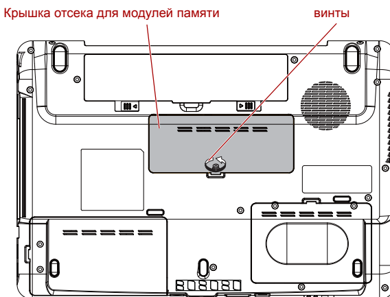
Рисунок 8-7 Устанавливаем крышку отсека для модулей памяти
