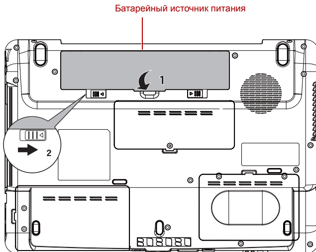
Рисунок 6-3 Установка батарейного источника питания
