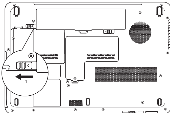
Рисунок 6-1 Высвобождение батарейного источника питания (1)
