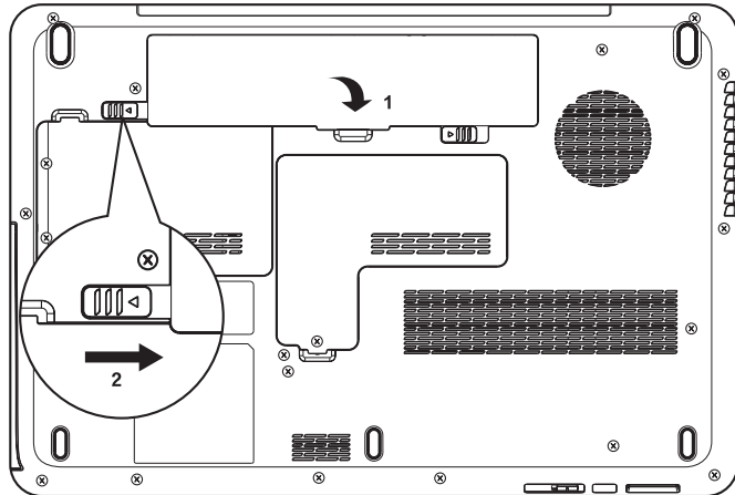
Рисунок 6-3 Установка батарейного источника питания
