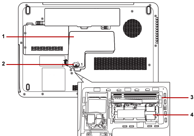
Рисунок 8-4 Снимаем крышку отсека для модулей памяти
