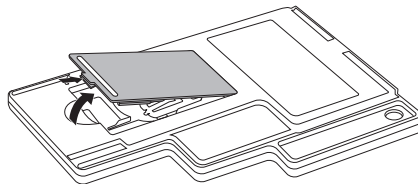
Рисунок 2-16 Открытие крышки батарейного отсека
