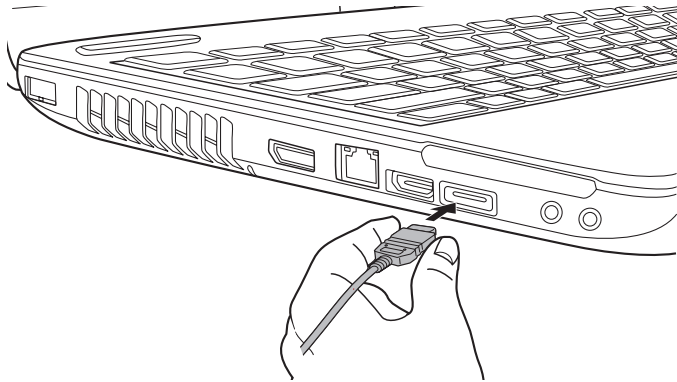
Рисунок 8-8 Подсоединение кабеля eSATA к порту USB (комбинированному порту eSATA)
