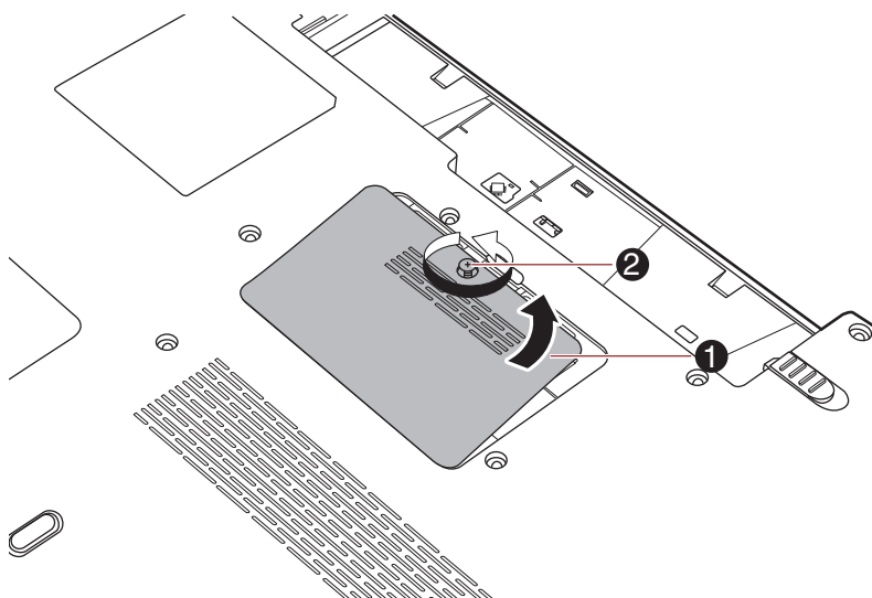
Рисунок 3-3 Снятие крышки отсека модулей памяти
