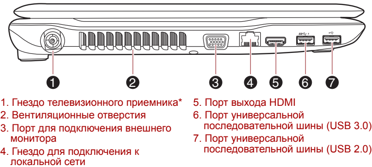
Рисунок 2-3 Левая сторона компьютера
