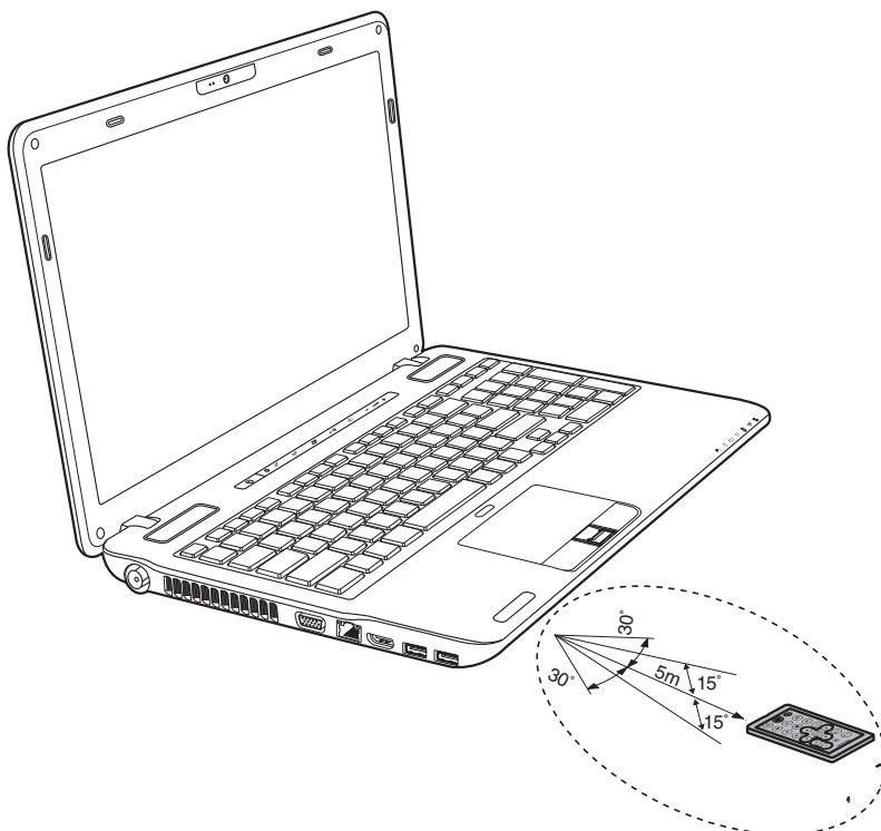
Рисунок 2-11 Радиус действия пульта дистанционного управления
