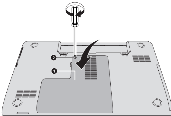
1. Крышка отсека модулей памяти 2. Винт
