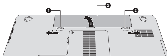
Рисунок 4-6 Высвобождение батарейного источника питания (2)
